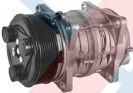
68618 New TM15 8 Groove 24 Volt Pulley Dia.: 4-11/16 Coil Clock: Wire Lead Seltec: 10355236, 48845236
