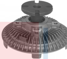
36980 REV Standard Duty Jeep (06-87) Chrysler: 68064284AA, 68064764AA, 68065080AA AMC: 52028327
