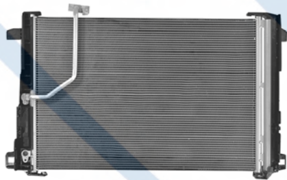
40312 Parallel Flow Mercedes (14-08) Mercedes Benz: 2045000654
