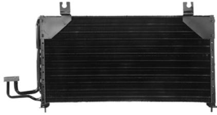
40666 Parallel Flow Kia (01-98) Kia: 1K2A161480A
