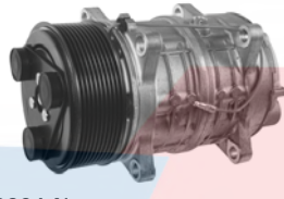
68621 New TM16 10 Groove 24 Volt Pulley Dia.: 4-11/16 Coil Clock: Wire Lead Seltec: 10356551
