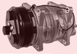
68623 New TM15HD 6 Groove 12 Volt Pulley Dia.: 4-11/16 Coil Clock: Wire Lead Seltec: 10355218, 48845218
